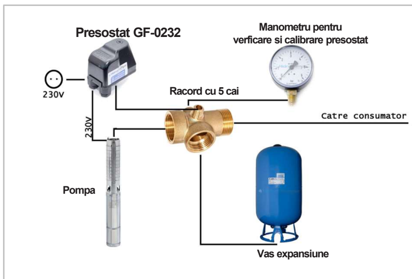
Schema montaj presostat in sistem hidrofor
